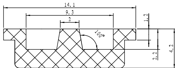
剖面 A-A
