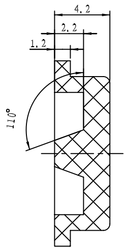
剖面 A-A
