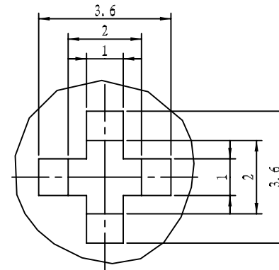
剖面 D-D
