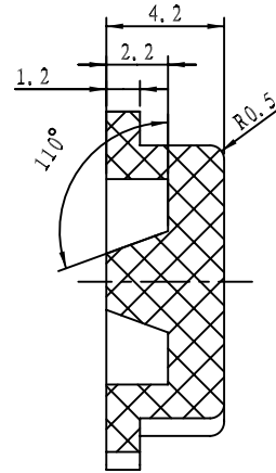
剖面 D-D
