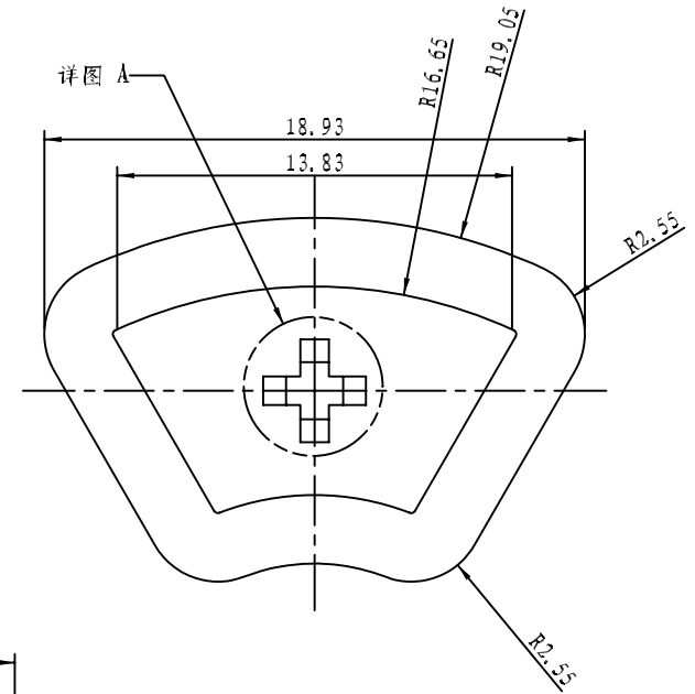
此面为顶杆面
