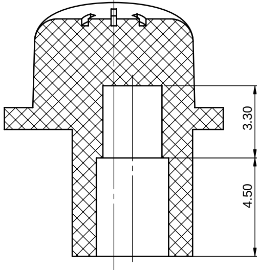
剖面 A-A
