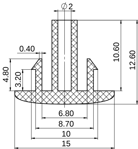
剖面 A-A
