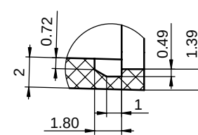
局部视图 F 比例 4:1
