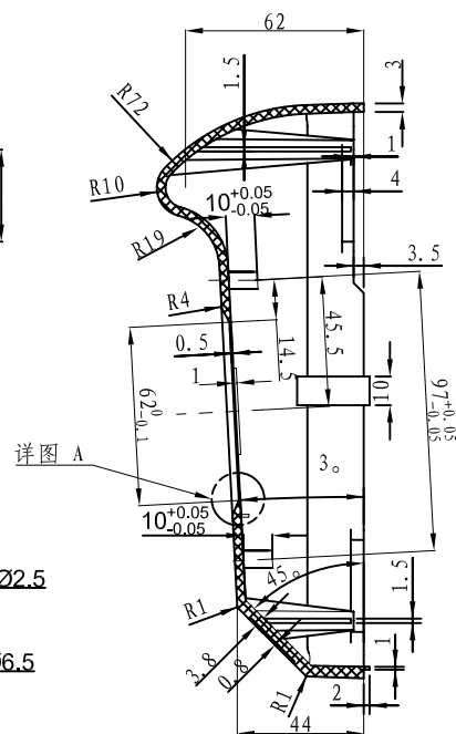
剖面 A-A
