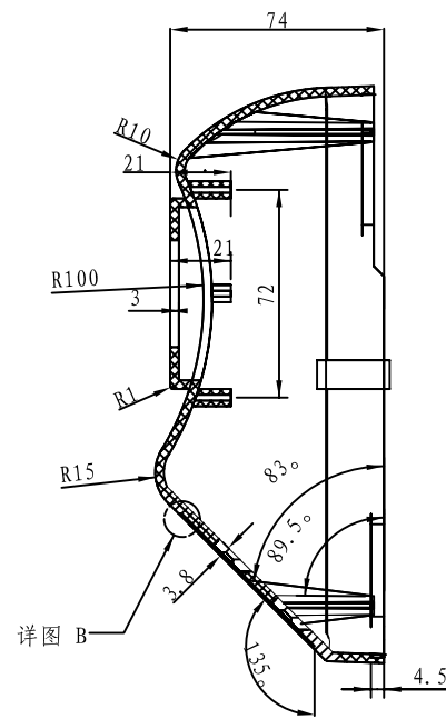
剖面 B-B
