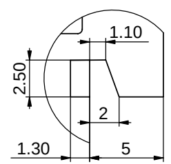
局部视图 J 比例 4:1
